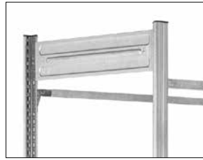
Aussteifungstraversen geben Stabilität und dienen auch zur Bodenaufgabe. Die Anzahl der Traversen richtet sich nach der Regalhöhe.
